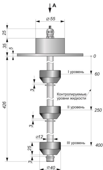
Габаритный чертеж
