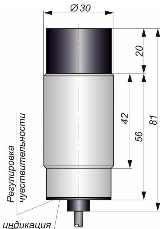
Габаритный чертеж
