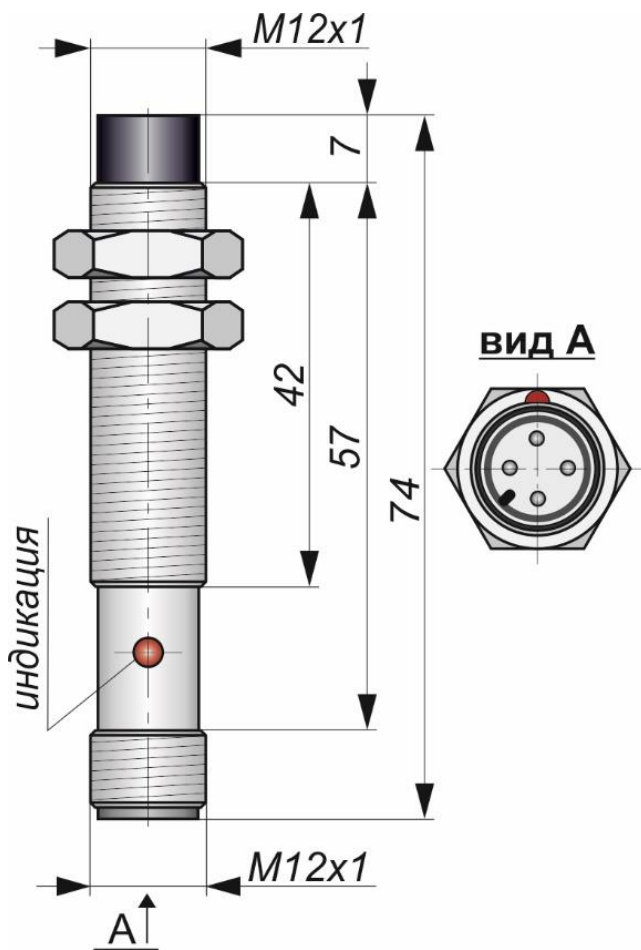
Габаритный чертеж
